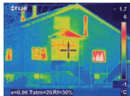
Die Thermografie macht die thermischen Schwachstellen mangelhafter Fensterfugen und den daraus resultierenden Wärmeverlust schnell deutlich.
