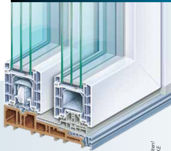
Ein Hebe-Schiebeflügel und zwei Festverglasungen
